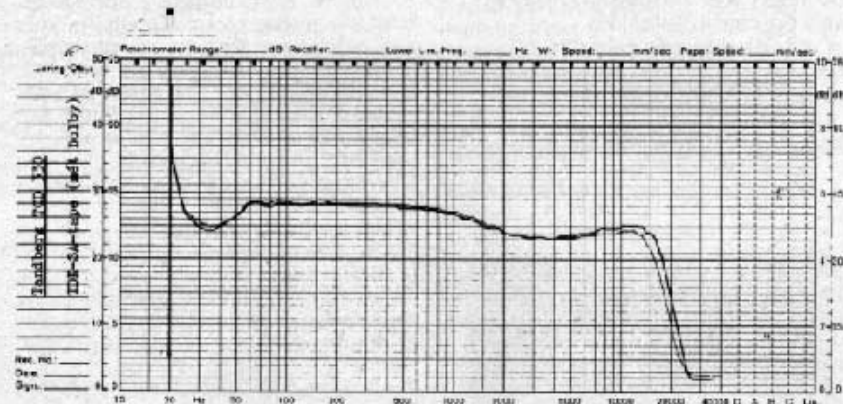
Dezelfde karakteristiek op TDK-SA band met en zonder dolby.
