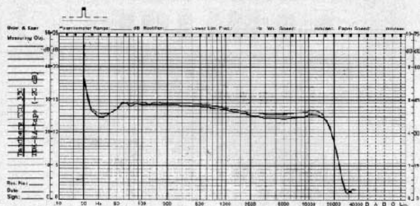
Over-all karakteristiek opgenomen op TDK-SA band.
